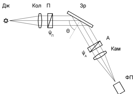
Рис. 1. Схема експерименту. Дж – джерело випромінювання, Кол – коліматорний об'єктив, П – поляризатор, Зр – зразок, А – аналізатор, Кам – камерний об'єктив, ФП – фотоприймач.
