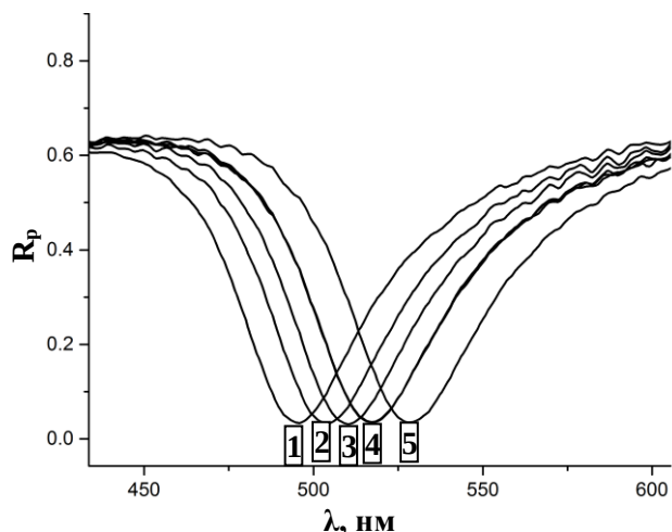
Рис.1. Залежності коефіцієнта відбиття р-поляризованого світла від довжини хвилі (нм) для зразка 1 при різних кутах падіння. Криві: 1, 2, 3, 4, 5 відповідають кутам падіння: 48^\circ , 47,7^\circ , 47,5^\circ , 47,3^\circ , 47^\circ .
