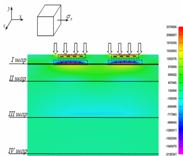
Рис.5. Поле напружень \sigma_x у перерізі дорожнього покриття з розшаруванням
