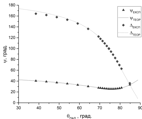
Рис. 2. Кутові залежності еліпсометричних параметрів \psi та \Delta для зразка Ti#4. Точки – експериментальні дані, лінії – теоретичні розрахунки.
