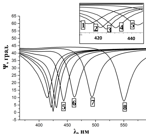
Рис.4. Залежності кута відновленої лінійної поляризації в градусах від довжини хвилі (нм) для зразка 3 при різних кутах падіння. Криві: 1, 2, 3, 4, 5, 6, 7, 8 відповідають кутам падіння: 60^\circ , 57,5^\circ , 56,5^\circ , 55^\circ , 52,5^\circ , 50^\circ , 47,5^\circ , 45^\circ .
