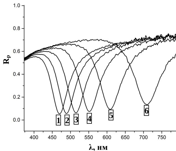
Рис.2. Залежності коефіцієнта відбиття р-поляризованого світла від довжини хвилі (нм) для зразка 2 при різних кутах падіння. Криві: 1, 2, 3, 4, 5, 6 відповідають кутам падіння: 50^\circ , 49^\circ , 48^\circ , 47^\circ , 46^\circ , 45^\circ .
