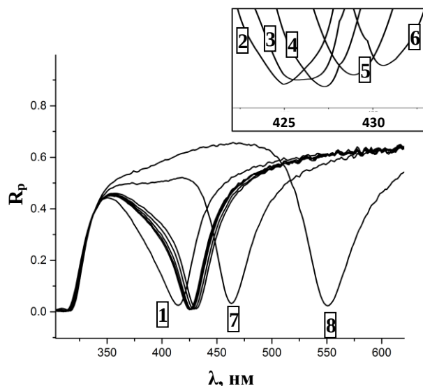
Рис.3. Залежності коефіцієнта відбиття р-поляризованого світла від довжини хвилі (нм) для зразка 3 при різних кутах падіння. Криві: 1, 2, 3, 4, 5, 6, 7, 8 відповідають кутам падіння: 60^\circ , 56,5^\circ , 56,3^\circ , 56^\circ , 55,5^\circ , 55^\circ , 50^\circ , 45^\circ .
