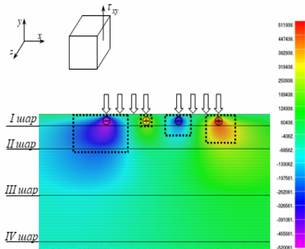
Рис.6. Розподіл дотичних напружень \tau_{xy}
