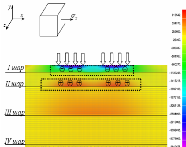
Рис.4. Поле напружень \sigma_x у перерізі дорожнього покриття
