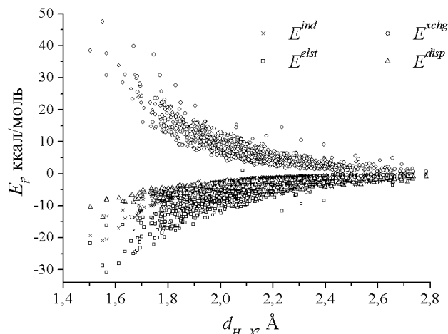
Рис. 4. Залежність внесків електростатичної ( E^{elst} ), дисперсійної ( E^{disp} ), індукційної ( E^{ind} ) та обмінної ( E^{xchg} ) взаємодії до загальної енергії взаємодії молекул воднево-зв'язаного комплексу від відстані d_{H...X} між атомом водню, здіяним у водневому зв'язку, та атомом-акцептором протона
