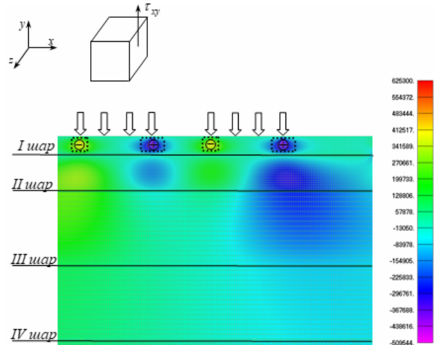
Рис.7. Розподіл дотичних напружень \tau_{xy} у покритті з розшаруванням
