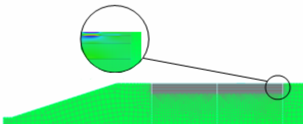
Рис.3. Скінченно-елементна модель перерізу дорожнього масиву
