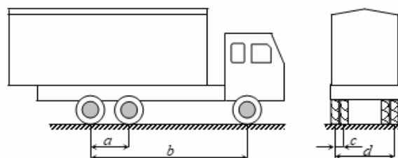
Рис.1. Геометрична схема розташування коліс тривісного автомобіля
