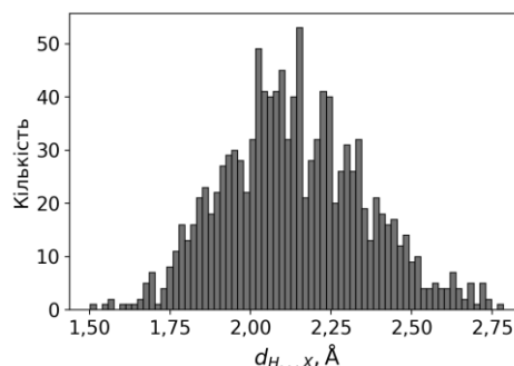
Рис. 1. Розподіл воднево-зв'язаних комплексів за відстанню d_{H...X} між атомом водню, задіяним у водневому зв'язку, та акцептором протона
