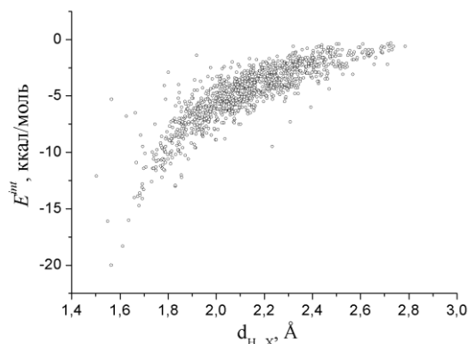
Рис. 2. Залежність енергії E^{int} взаємодії молекул воднево-зв'язаного комплексу від відстані d_{H...X} між атомом водню, задіяним у водневому зв'язку, та атомом-акцептором протона
