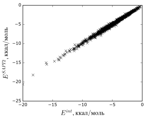
Рис. 3. Взаємозв'язок між величинами енергії взаємодії молекул воднево-зв'язаного комплексу, знайдених супрамолекулярним методом ( E^{int} ) та з використанням адаптованої до симетрії теорії збурень ( E^{SAPT2} )
